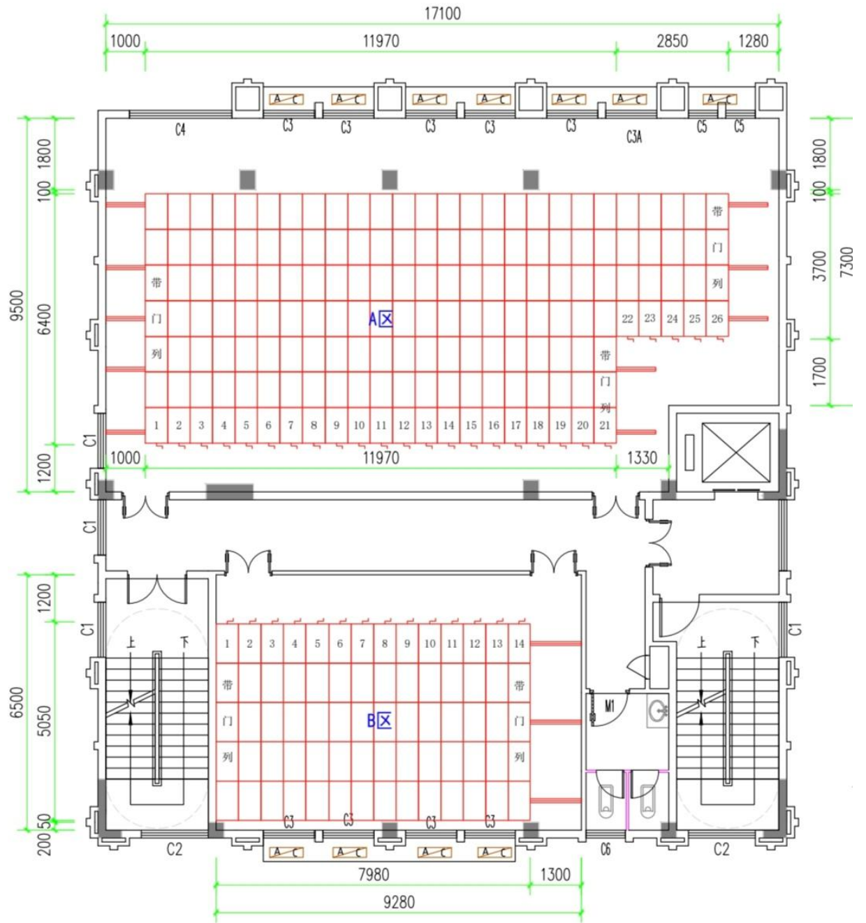
4~5层档案室密集柜布置平面图
