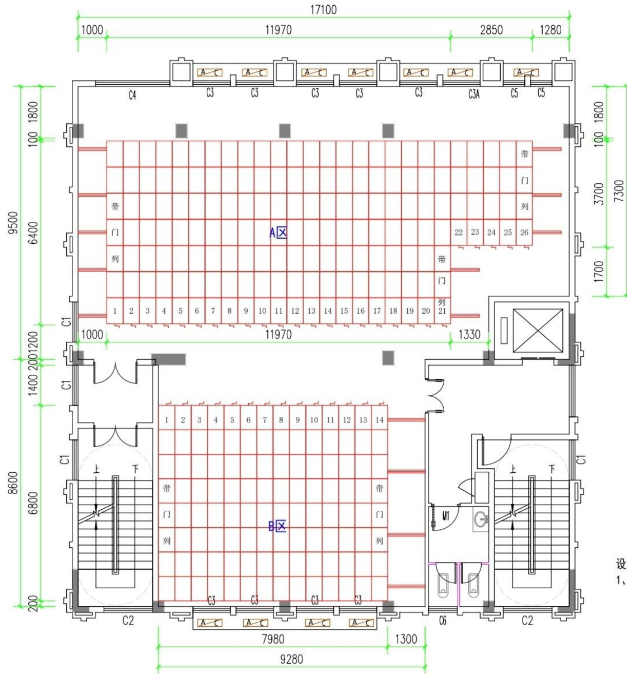
6层档案室密集柜布置平面图
